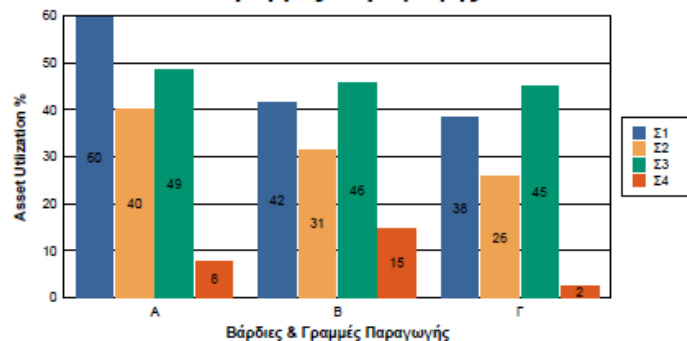
Asset Utilization - Τρέχοντος Έτους / Βάρδιες & Γραμμές Παραγωγής
