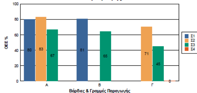
OEE - Τρέχουσες Ημέρες / Βάρδιες & Γραμμές Παραγωγής
